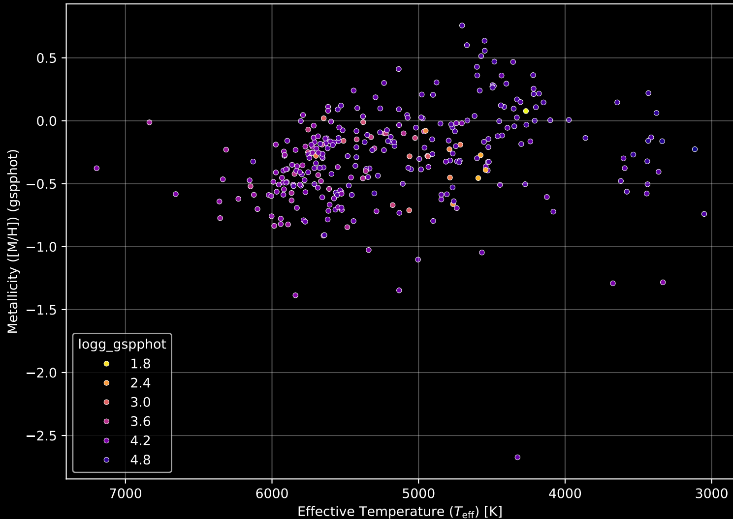
APOGEE DR17 Field: [sgr_tidal13] Stellar Population Parameters (n= 305)
